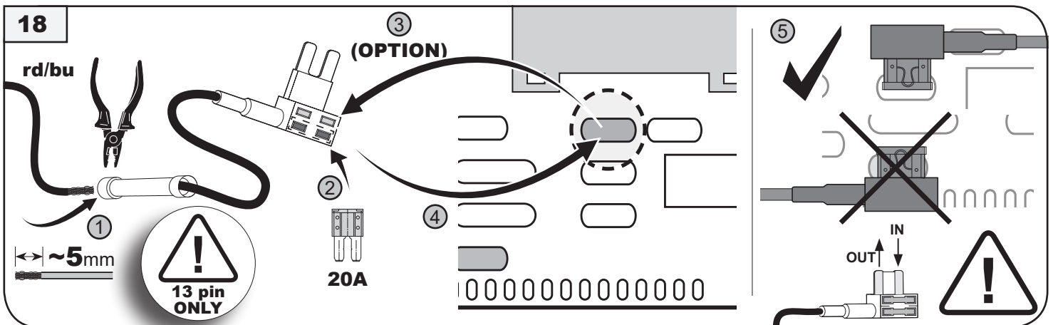
Sicherung 20A → E-Satz rd/bu → Sicherungskasten F05 fuse 20A → e-kit rd/bu → fusebox F05
