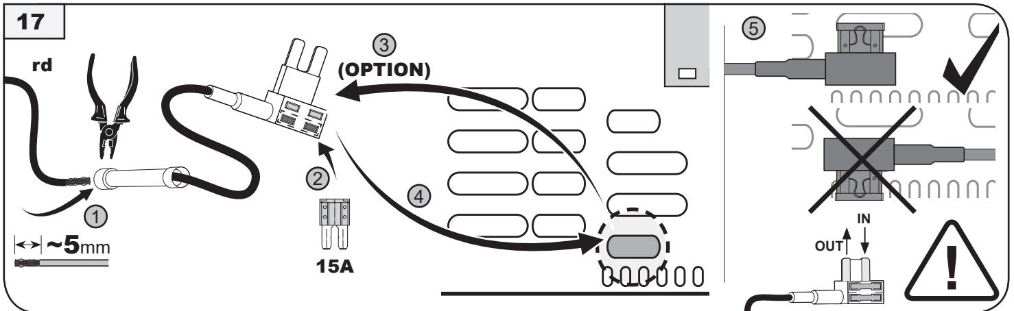
Sicherung 15A → E-Satz rd → Sicherungskasten F24 fuse 15A → e-kit rd → fusebox F24
