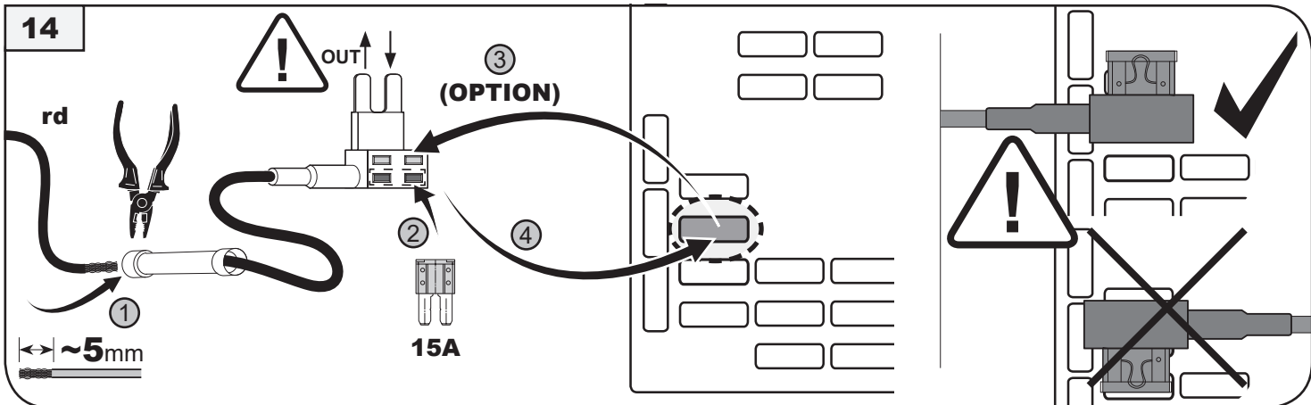
Sicherung 15A → E-Satz rd → Sicherungskasten fuse 15A → e-kit rd → fusebox
