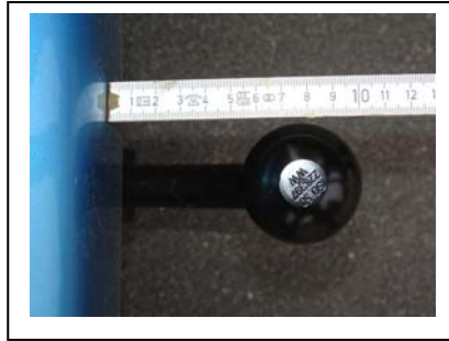
Abstand Stoßfänger – Kugelkopf
